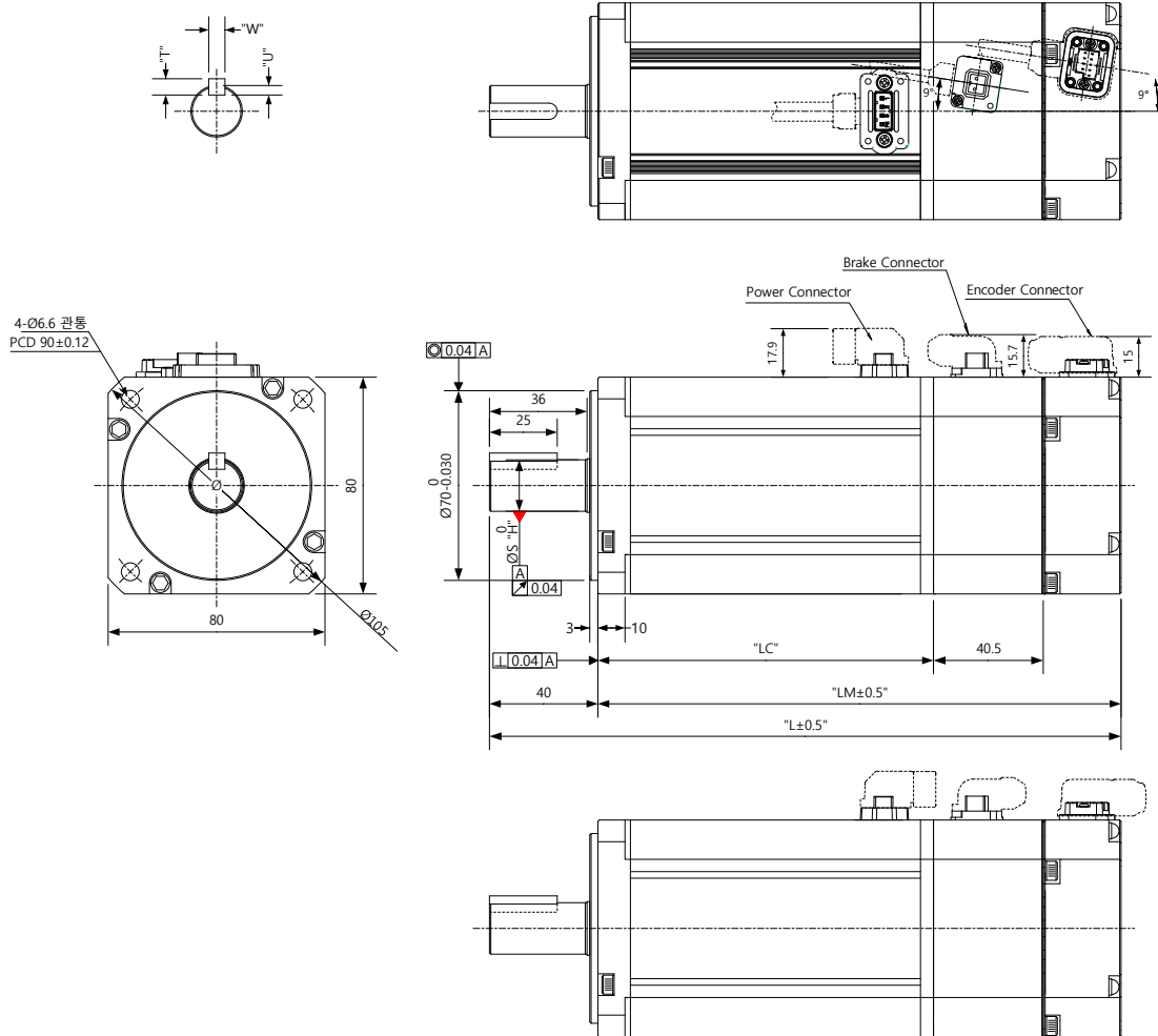
<Cable 인출 방향이, 축 반대 방향일 경우>
