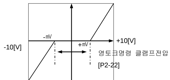
영토크명령 클램프전압 [P2-22] = Not 0[mV]
