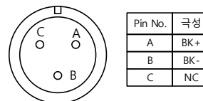
Plug : MS3102A14-7P
