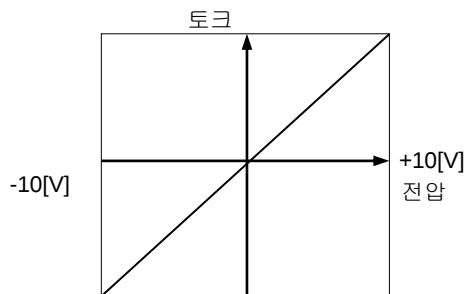
영토크명령 클램프전압 [P2-22] = 0
