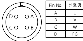
Plug : MS3102A32-17P
