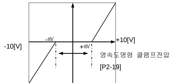
영속도명령 클램프전압 [P2-19] = Not 0[mV]
