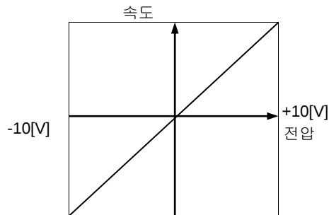
영속도명령 클램프전압 [P2-19] = 0
